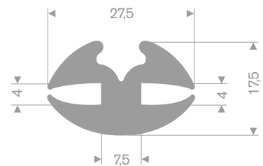
213.00.238GR TPE 70° Shore black roll length 30 meter
