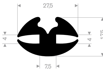
213.00.238 EPDM 70° Shore black roll length 50 meter
