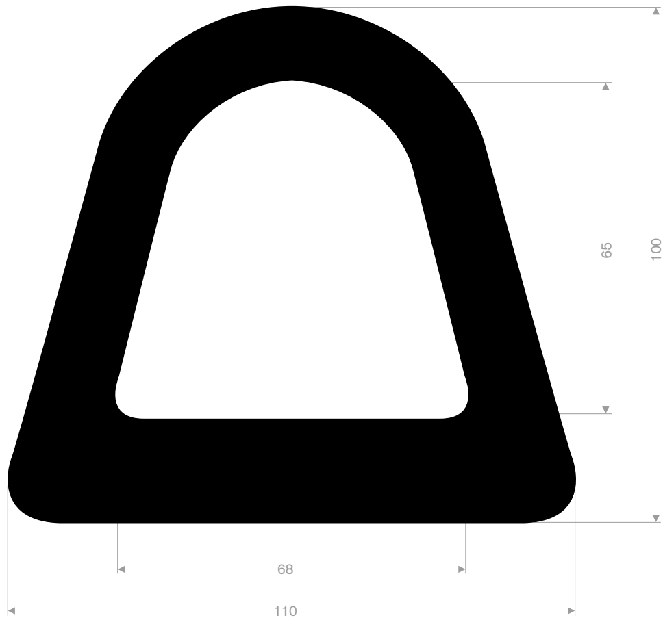
215.11.010 EPDM 70° Shore black roll length 12,50 meter
