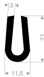
211.00.224 EPDM 70° Shore black roll length 50 meter
