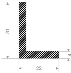
225.01.125 EPDM 15° Shore black roll length 25 meter
