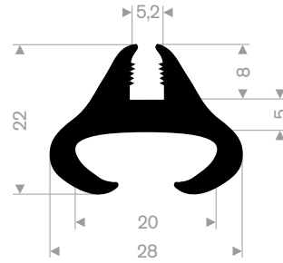
213.00.816 EPDM 70° Shore black roll length 20 meter
