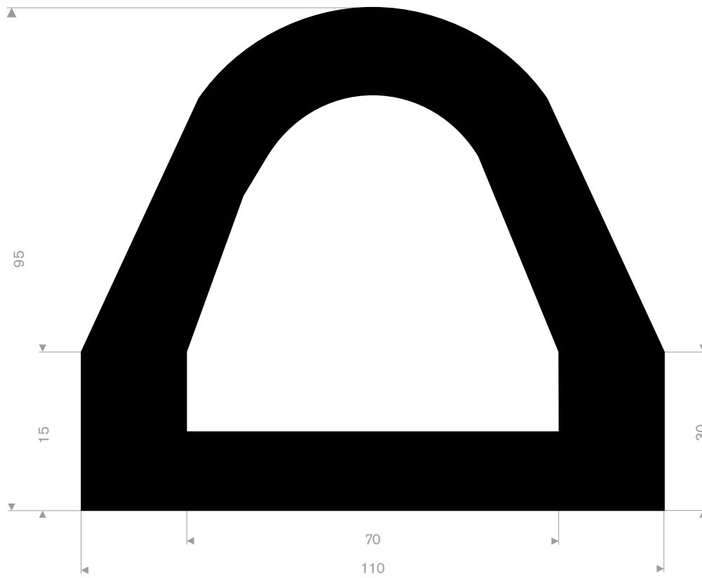
215.01.195 EPDM 70° Shore black roll length 5 meter
