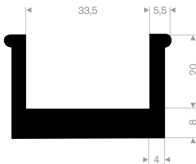
211.08.222 EPDM 70° Shore black roll length 25 meter
