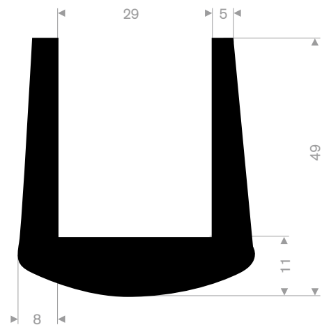
211.05.511 EPDM 70° Shore black roll length 25 meter
