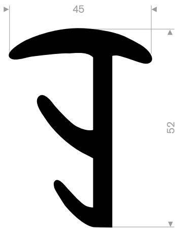
216.05.760 EPDM 70° Shore black roll length 25 meter
