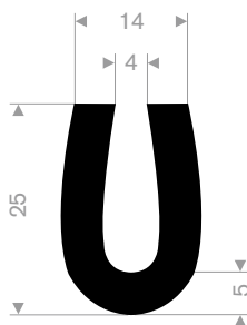
211.04.510 EPDM 70° Shore black roll length 30 meter
