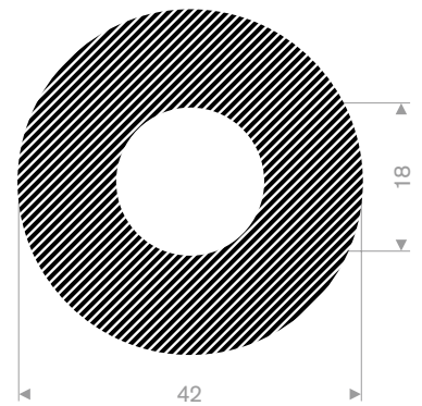
222.01.842 EPDM 15° Shore black roll length 10 meter
