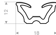
219.01.204 EPDM flocked roll length 30 meter
