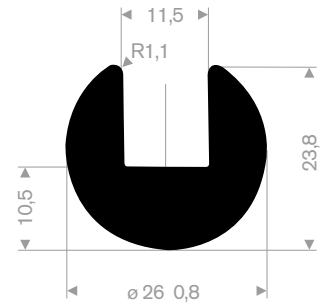
211.04.385 EPDM 70° Shore black roll length 50 meter
