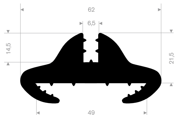
213.00.866 EPDM 70° Shore black roll length 25 meter
