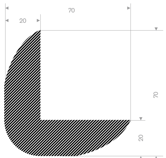
225.01.170 EPDM 15° Shore black roll length 10 meter
