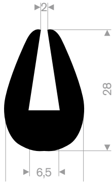
211.00.565 EPDM 70° Shore black roll length 50 meter
