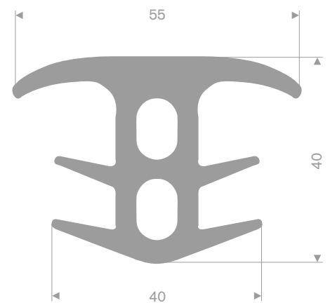
black 216.05.801GR EPDM 70° Shore grey roll length 15 meter
