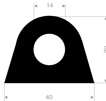
215.14.031 EPDM 65° Shore black roll length 20 meter
