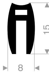
211.09.008 EPDM 65° Shore black roll length 25 meter
