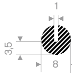
221.01.108 EPDM 15° Shore black roll length 100 meter
