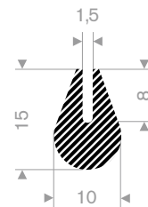
221.00.110 EPDM 15° Shore black roll length 100 meter
