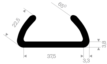
211.08.004 EPDM 70° Shore black roll length 50 meter
