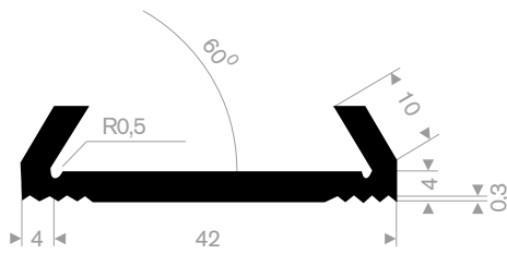
211.08.011 EPDM 70° Shore black roll length 50 meter
