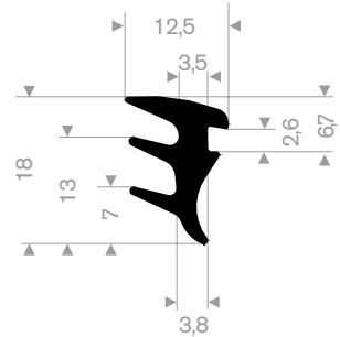
216.03.557 EPDM 65° Shore black roll length 100 meter
