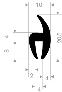
212.00.048 EPDM 70° Shore black roll length 50 meter
