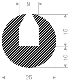
221.01.825 EPDM 15° Shore black roll length 30 meter
