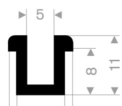
211.01.026 EPDM 70° Shore black roll length 30 meter
