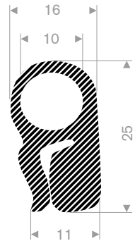
225.00.083 EPDM 15° Shore black roll length 30 meter
