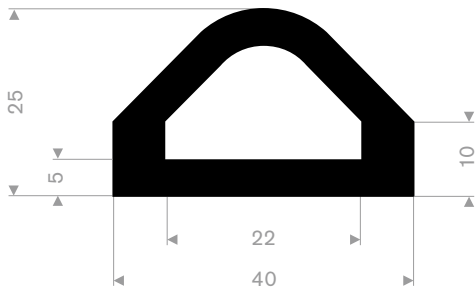
215.04.025 EPDM 70° Shore black roll length 5 meter
