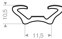
219.01.201 EPDM flocked roll length 30 meter
