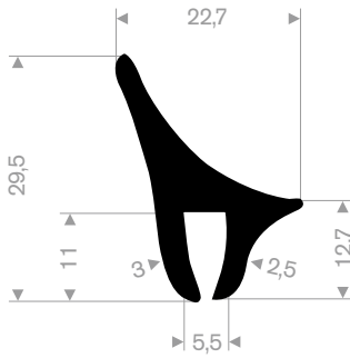
211.00.233 EPDM 70° Shore black roll length 50 meter
