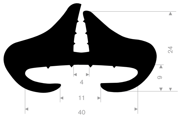
213.00.850 EPDM 70° Shore roll length 30 meter
