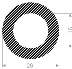
222.01.626 EPDM 15° Shore black roll length 50 meter
